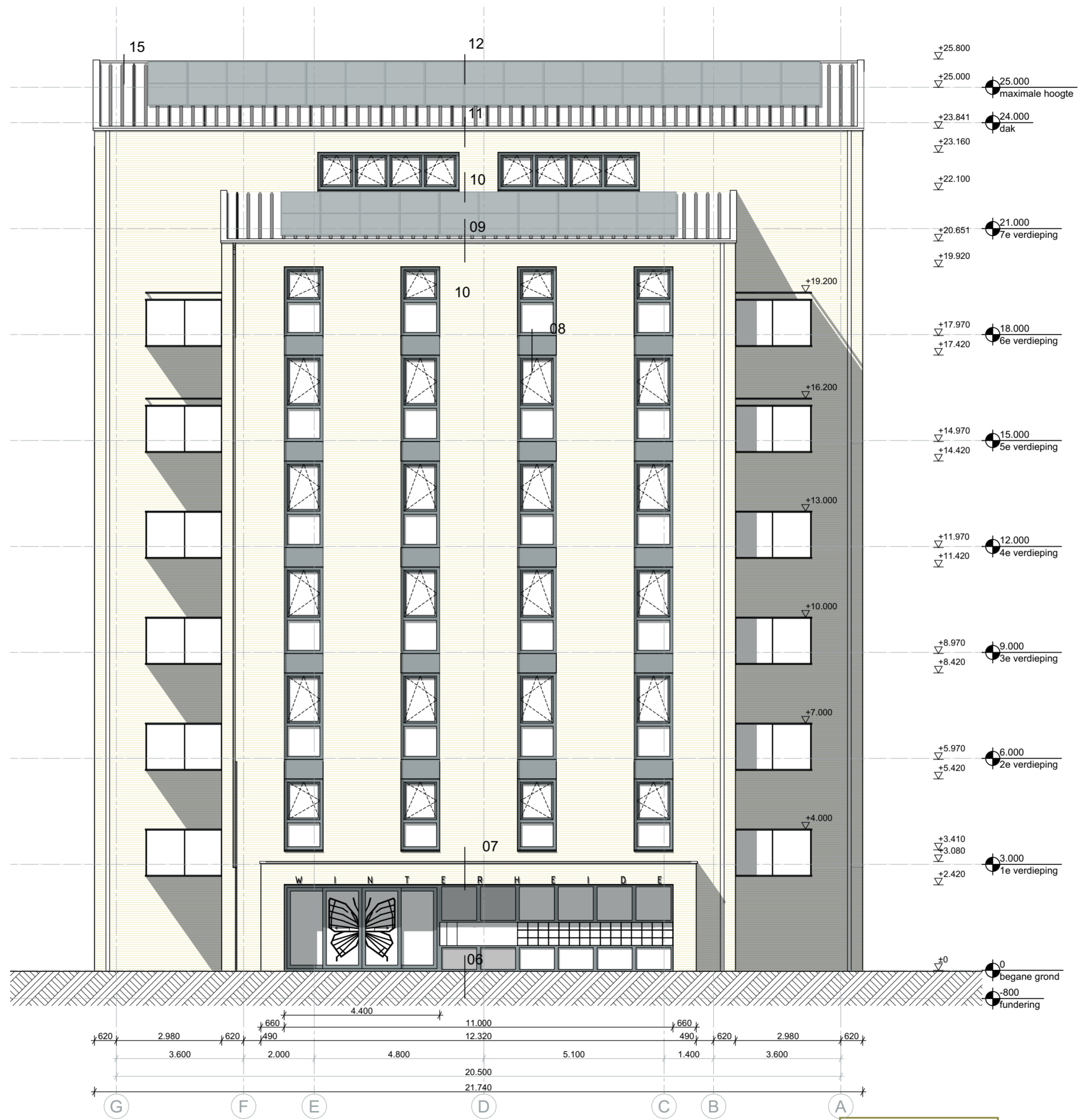
gevel noordoost
